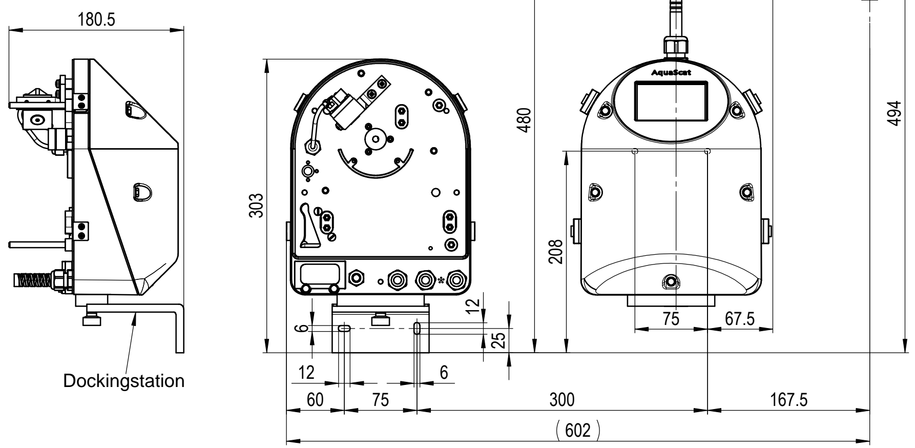
Montage Gerät für Wartung auf Dockingstation Mounting of instrument for maintenance on dockingstation
